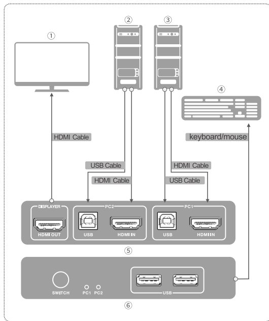
①TV ②PC2 ③PC1 ④键盘鼠标 ⑤KVM切换机正面 ⑥KVM切换机反面
